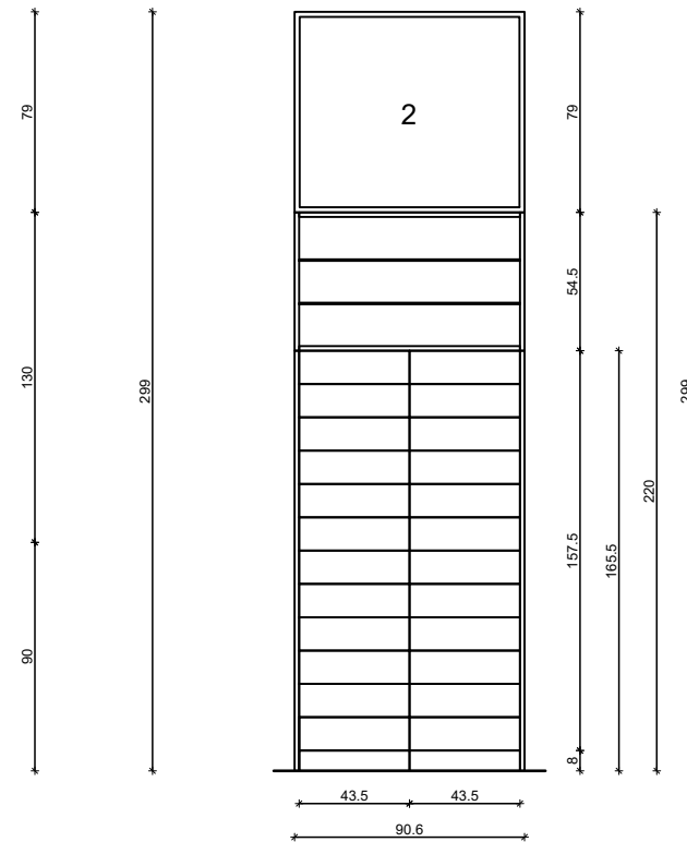
Presjek P2-P2
